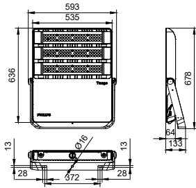
BVP384 LED528/857 490W 220-240V S6 L GC
