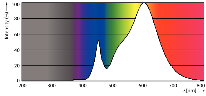
LEDspot MAS 37W E27 PAR30L 830 15D ND
